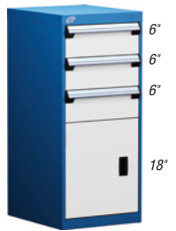
3 drawers / 1 door
